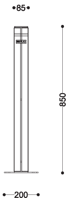
Rzut z frontu
