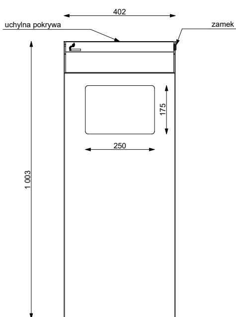
Rzut z frontu
