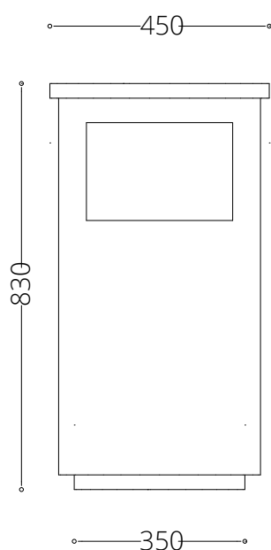
Rzut z frontu
